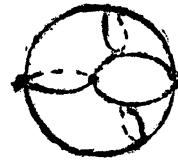
B(X)/S(X) \simeq S/A
