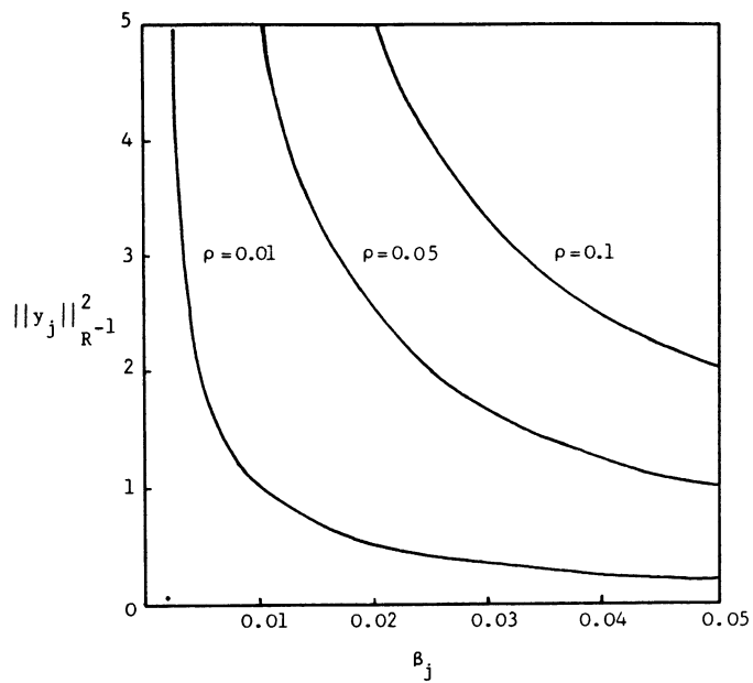
Figure 1. — Pourcentage maximum d'augmentation d'une valeur propre lorsque le poids p_j augmente jusqu'à \tilde{p}_j .
