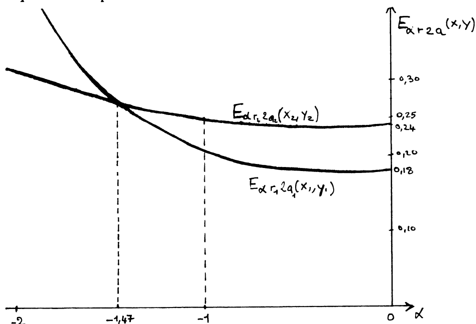
Graphique G5 : Evolution des écarts-type E_{\alpha r 2a}
