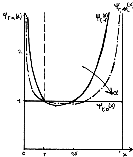
Cas \alpha \leq 0
