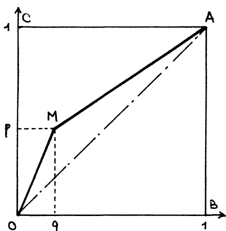
Cas de figure : p \geq q
