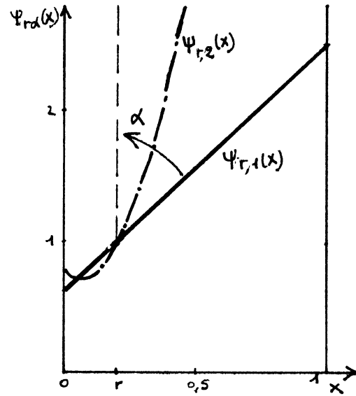
Cas \alpha \geq 1
