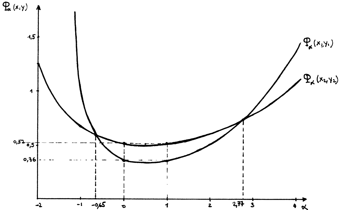
Graphique G2 : Évolution des indices \Phi_\alpha
