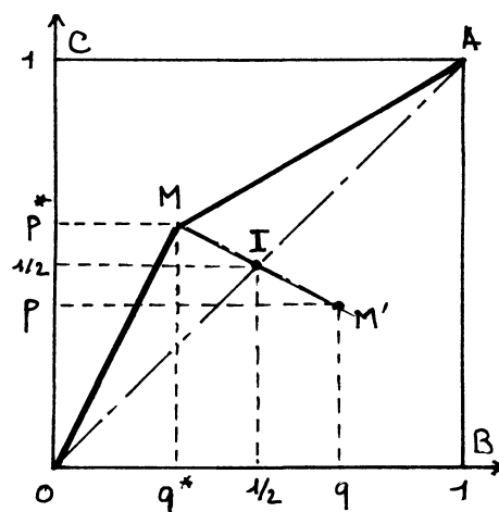
Cas de figure : p < q
