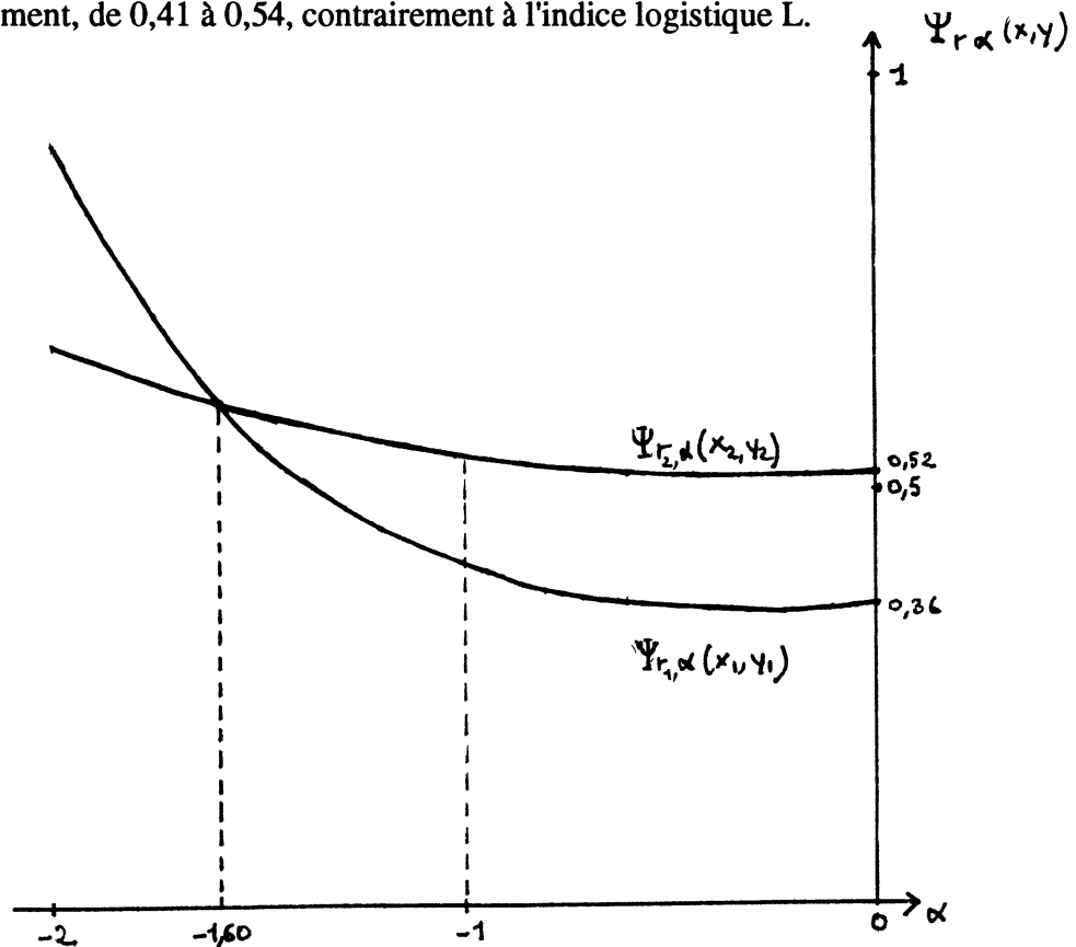
Graphique G4 : Évolution des indices \Psi_{r\alpha}
