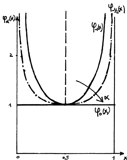
Cas \alpha \leq 0
