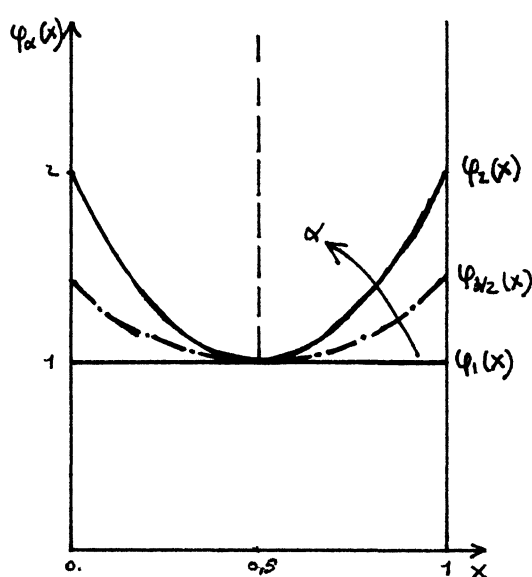
Cas \alpha \geq 1
