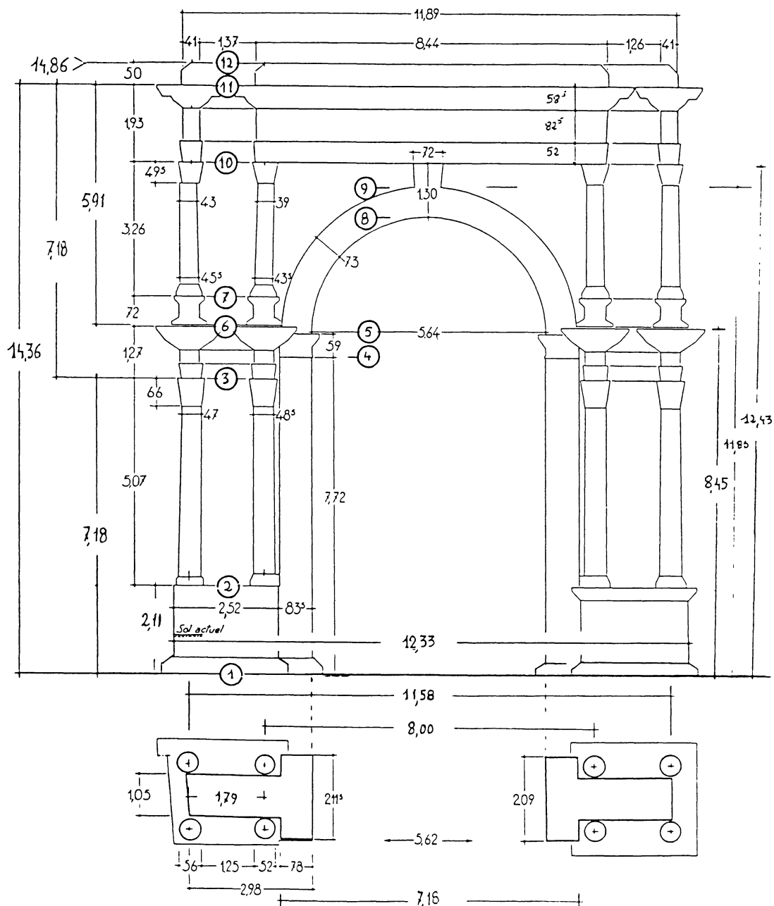
Figure 2 - Principales dimensions de l'arc
