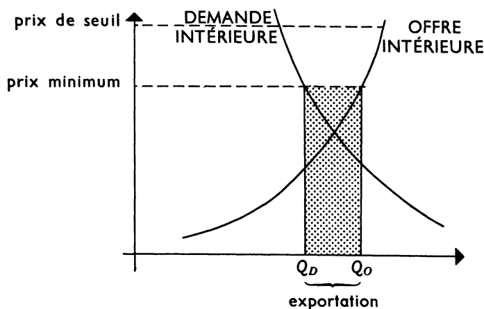
Graphique 2. Équilibre du marché en situation excédentaire
