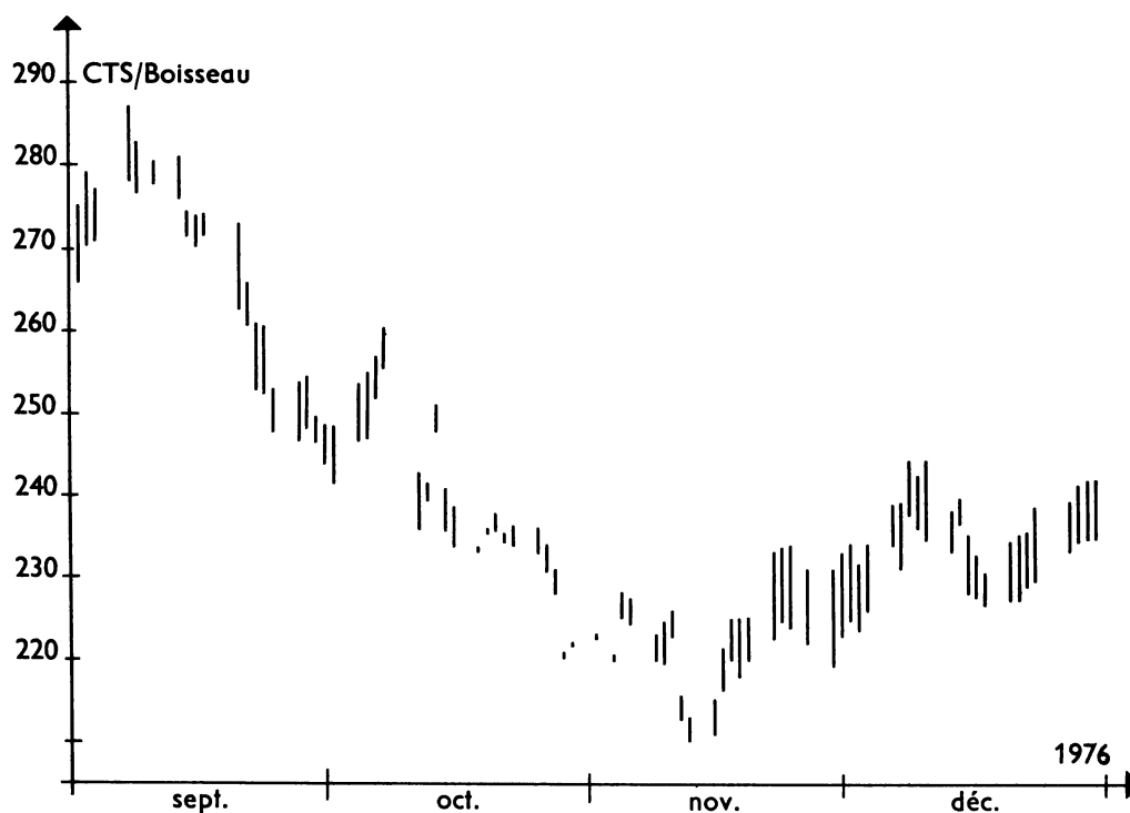
Graphique 3. Étendue statistique des fluctuations des prix du maïs, au comptant, sur la place de Chicago d'après les statistiques du Chicago Board of Trade (1977)
