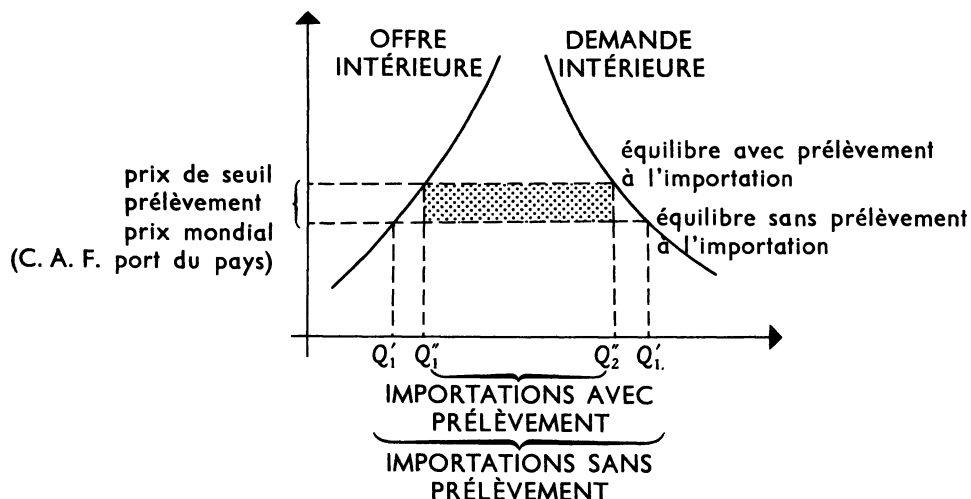
Graphique 1. Équilibre du marché en situation déficitaire avec, ou sans prélèvement à l'importation
