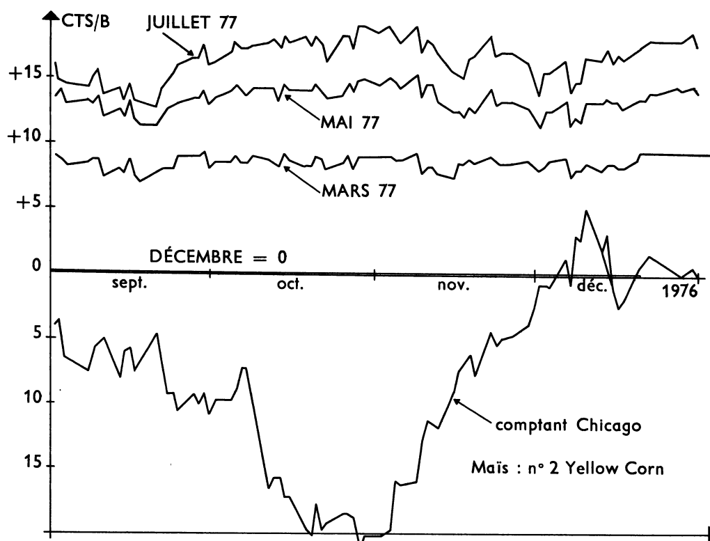
Graphique 4. Différences de prix au comptant et à terme, base 0 : prochaine échéance d'après les statistiques du Chicago Board of Trade (1977)
