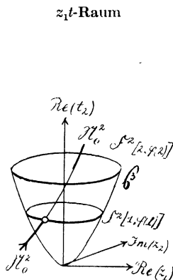
Fig. 2b. Der Schnitt von \mathfrak{H}^3 mit dem Raum \varphi_2 = 0 .
