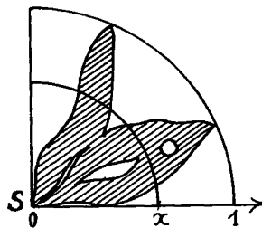
Figure 3: on a couvert de hachures le domaine des qualités que possède un individu i ; on convient d'attribuer à i la notion limite L parce que, des qualités situées à la distance x (sur un quart de cercle) il possède une part supérieure à (1-x) .
