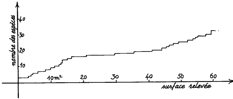
Figure 1: Courbe des relevés servant à définir un individu d'association; l'aire floristiquement homogène peut être prise entre 15 et 40m 2 environ.
