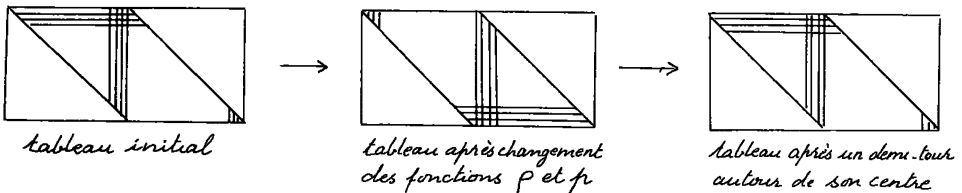
Figure 4 : Schéma des changements ; on a suggéré par des hachures les valeurs inégales des fonctions de densité p(x) et p(x) .
