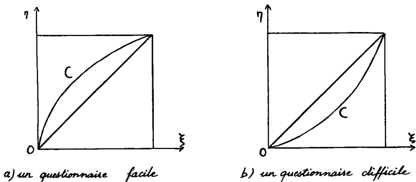
Figure 1 : deux exemples de courbe C
