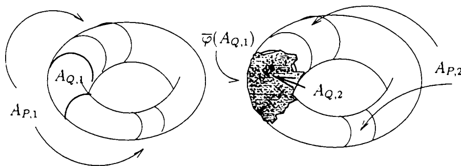
FIG. 13.2 - Applications entre tores.
