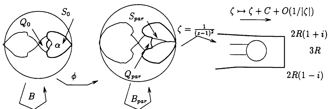
FIG. 7.11 - Définition de \phi .
