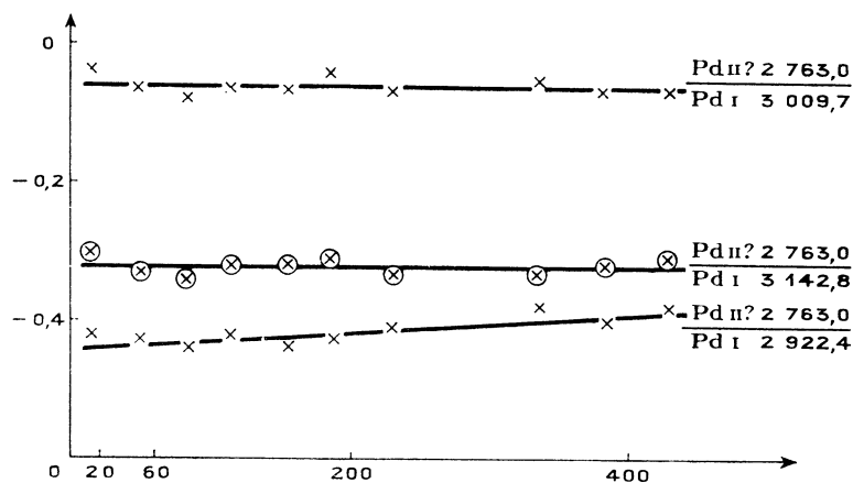
FIG. 9. — Comportement, en fonction du temps, de la raie Pd II? 2763,0 Å. En abscisse, temps en secondes, en ordonnée, log ( I_{\text{ét.}}/I_{\text{arc}} ).
