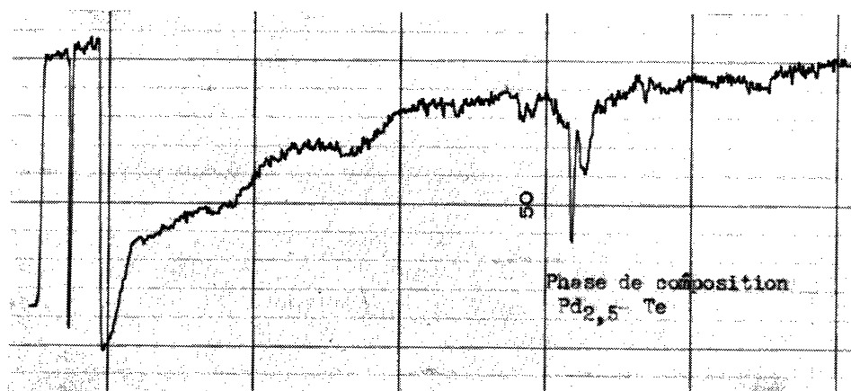
FIG. 23. — Coprécipité du palladium avec le tellure. Réduction par le sulfate d'hydrazine, en milieu chlorhydrique 0,5 N. \text{Te/Pd} = 5 .
