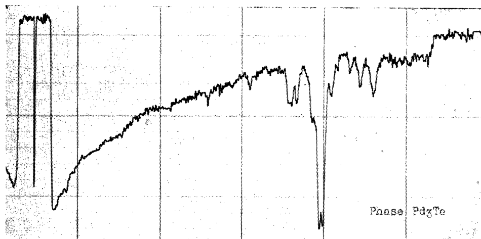
FIG. 19. — Coprécipité du palladium avec le tellure. Réduction par l'anhydride sulfureux, en milieu chlorhydrique 2 N. \text{Te/Pd} = 1/2 .
