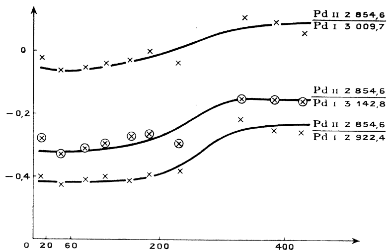
FIG. 8. — Renforcement, en fonction du temps, de la raie Pd II 2854,6 Å. En abscisse, temps en secondes; en ordonnée, log ( I_{\text{ét.}}/I_{\text{arc}} ).
