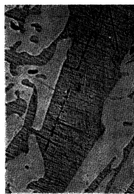
Photographies 11 et 12. — Alliage Al-Co à 10 % de Co, maintenu pendant 3 heures à la température de 680°, puis refroidi à l'air. Sections de lamelles d'Al 3 Co 2 dans un fond d'aluminium. Lumière naturelle (G = 50 X).
