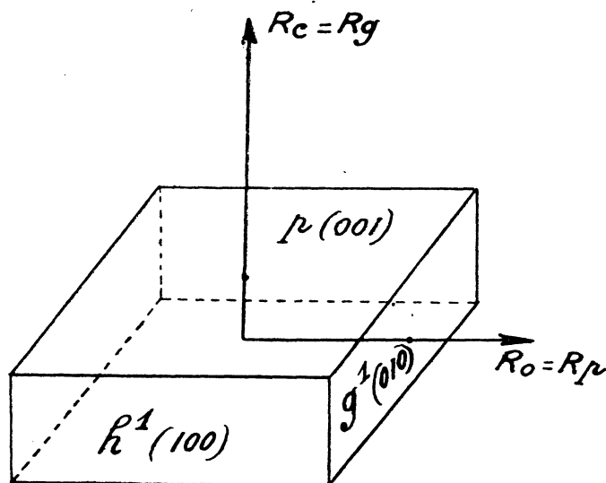
FIG. 15. — Répartition des pouvoirs réflecteurs dans le cristal \text{Al}^3\text{Ti} .
