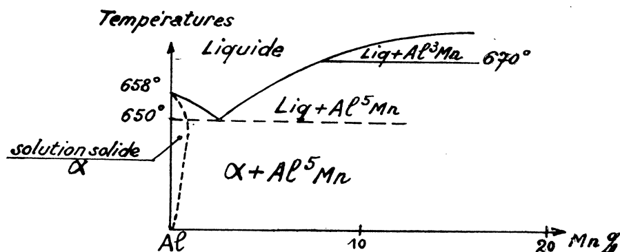
FIG. 16. -- Diagramme Al-Mn d'après Ishiwarara.
