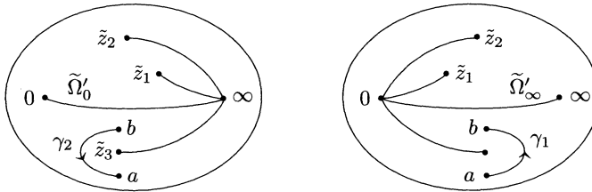
Figure 2. Domaine de définition de \tilde{X}^{(0)} (à gauche) et de \tilde{X}^{(\infty)} (à droite)
