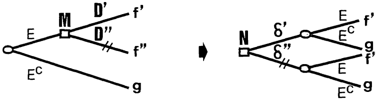
Figure — L'axiome d'indépendance A2 affirme que, préférant en M la décision D' à la décision D'', le Décideur doit en N préférer la décision \delta' à la décision \delta'' .
