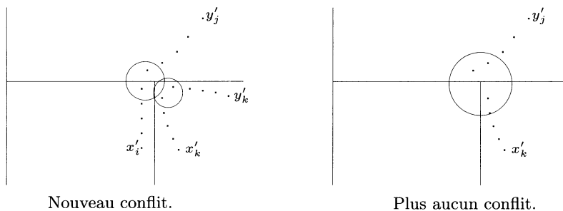
FIGURE 8. Le nombre de conflits est borné.
