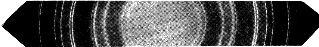
Aluminium 2 mg. recuit pendant 2 heures à 400° C.
