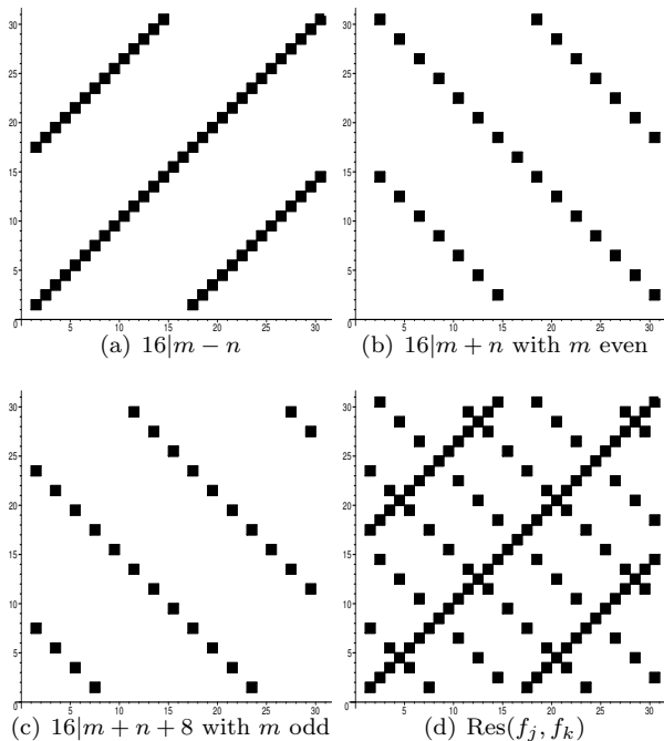
FIGURE 6. f = x^2 - 3x - 1
