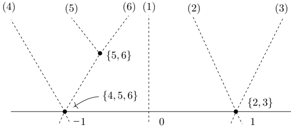
FIG. 1.1. L'arbre d'éclatements de l'exemple 1.6
