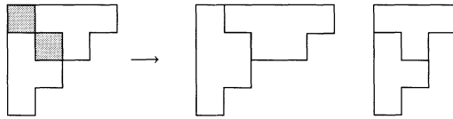
Figure 6. Puissances extérieures d'un carré symétrique ou extérieur
