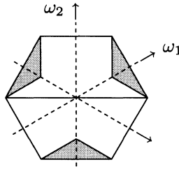
Figure 12. Le saturé du polygone C_{(2,1),2,3} .
