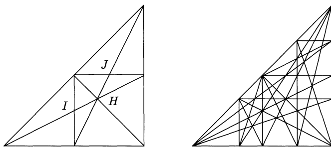
Figure 13. Constructions stabilisantes pour S^2\mathbb{C}^4 et S^3\mathbb{C}^4 .
