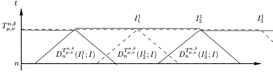
Figure 2. Étude du décalage d'amplitude induit par les interactions d'ordre \nu qui se produisent à l'intérieur du domaine D_n^{T_{\mu,\nu}^{n,\delta}}(I_p^1; I)
