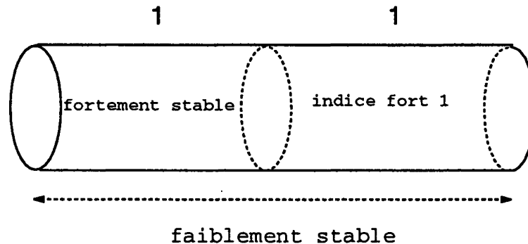
FIG. 1: Stabilité pour le domaine \mathcal{G}_a
