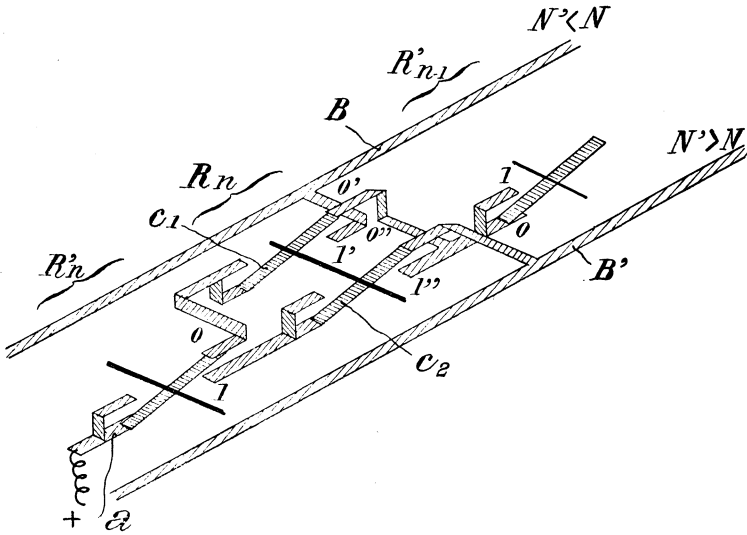
Fig. 11. — Schéma d'un comparateur.
