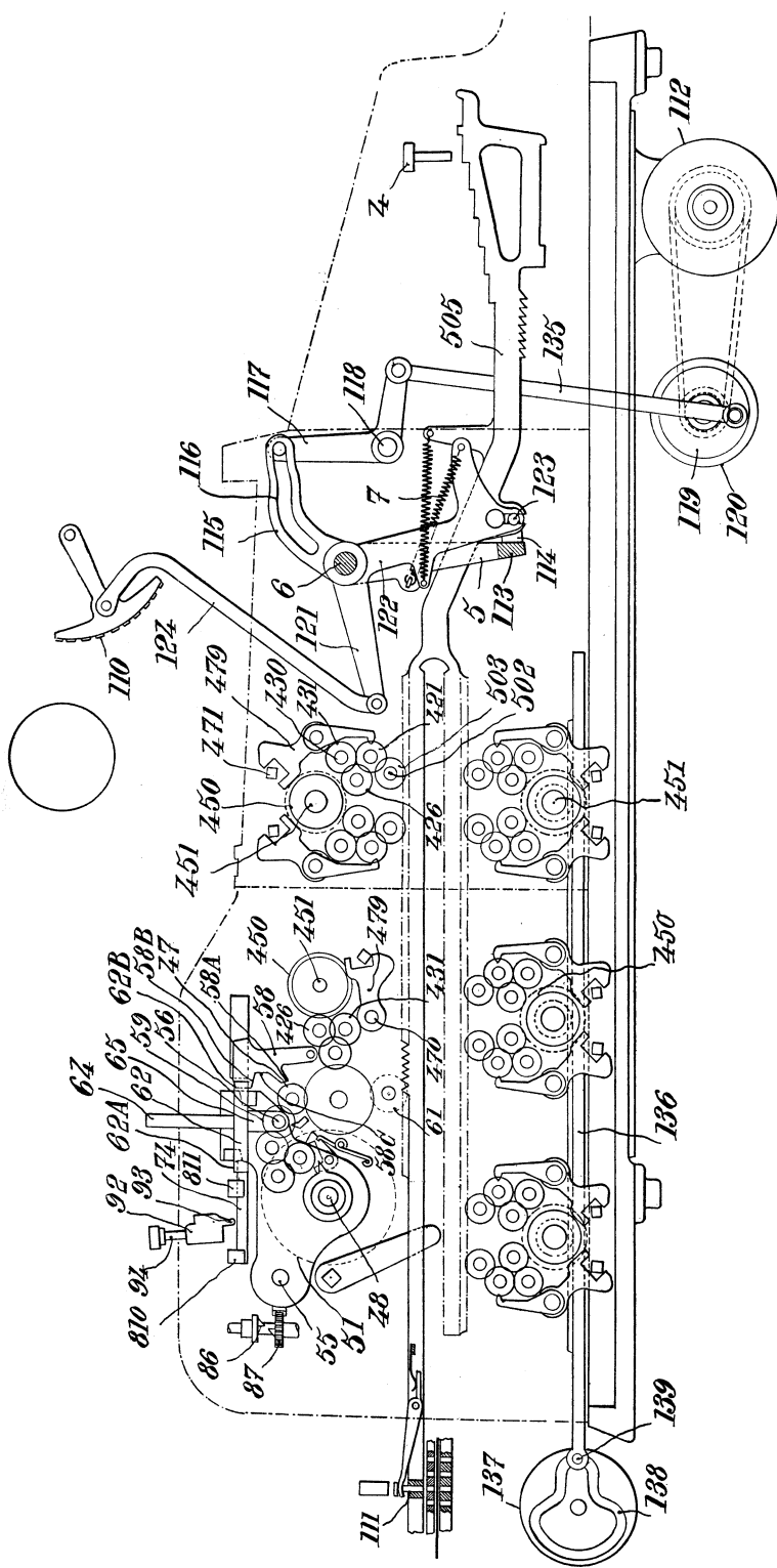
Fig. 4. — Vue d'ensemble d'une réalisation de la machine décimale.
