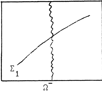
Cas A
