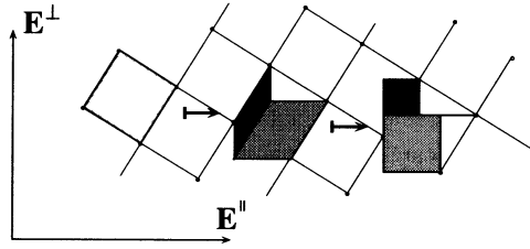
FIGURE 3. Une déformation itérative des arêtes du carré type mène au “pavage oblique”
