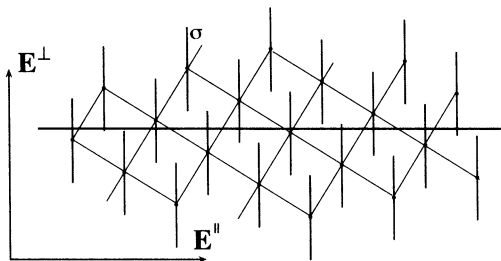
FIGURE 2. La construction canonique des pavages du type de Penrose en dimensions minimales
