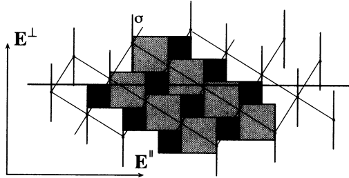
FIGURE 4. Le pavage oblique en dimensions minimales
