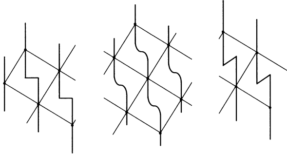
FIGURE 5. La “complétion” de la surface atomique doit obéir à une condition d’orientation relative : le troisième cas de figure ci-dessus fait apparaître le long du raccord oblique un “anti-atome” sans signification physique.
