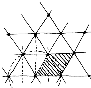
tore équilatéral
