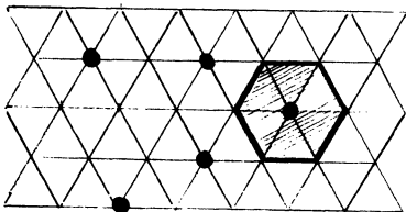
Fig.9 - Une configuration de points contribuant à h(n,D) .
