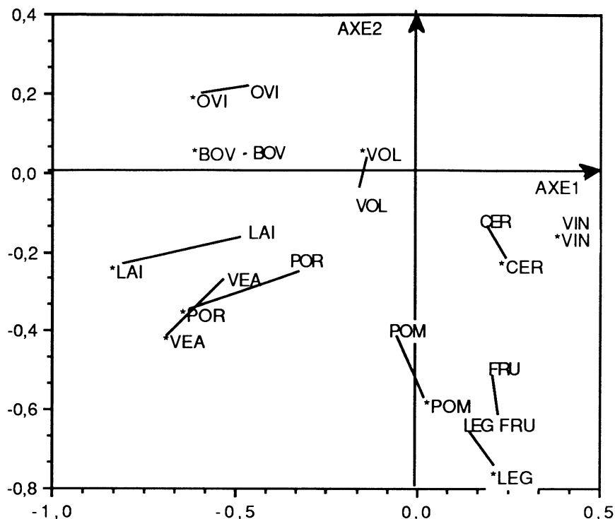
FIGURE 5 Plan 1-2 de l'A.F.D.L. * = variable résidu
