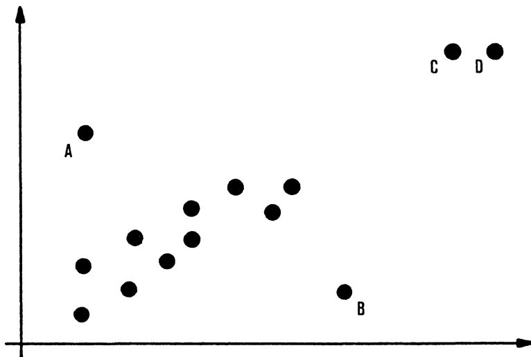
FIGURE 2.1. Données artificielles dans \mathbb{R}^2
