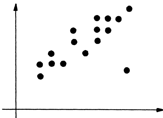
FIGURE 1.1. Données artificielles dans le plan
