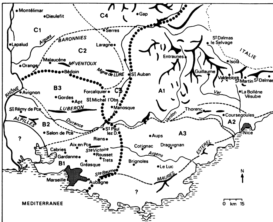
Figure 1. — Carte du Sud Est de la France et les 10 zones pluviométriques délimitées par la classification hiérarchique rassemblées en trois groupes A, B, C.
