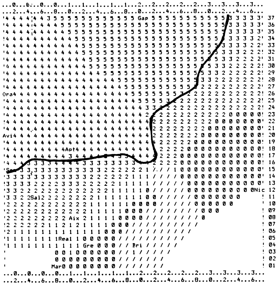
Figure 6. — C.P. 1 de la matrice de covariance des spectres de 12 séries mensuelles de précipitations.
