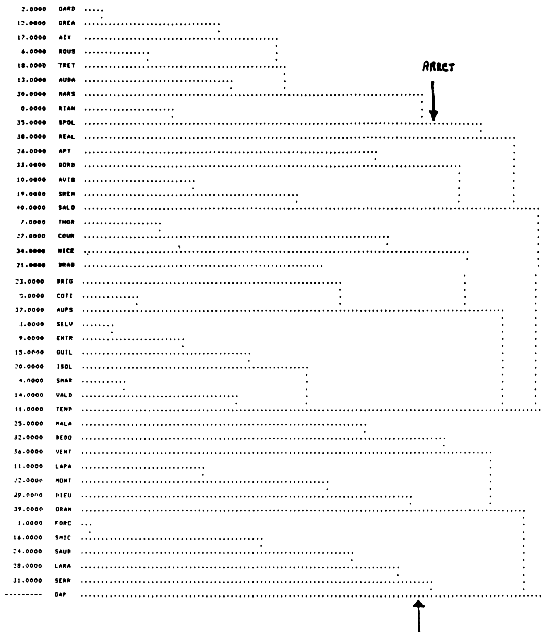
Figure 5. — Arbre de la classification hiérarchique des 42 séries de précipitations.
