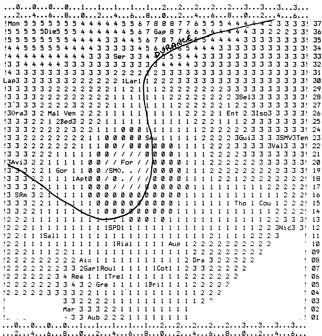
Figure 2. — Composante principale 1 des précipitations projetée sur la carte des 42 stations.
