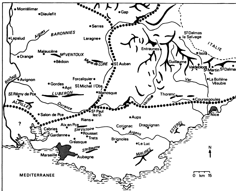
Figure 9. — Délimitation de 4 zones basées sur les 6 variables synthétiques.
