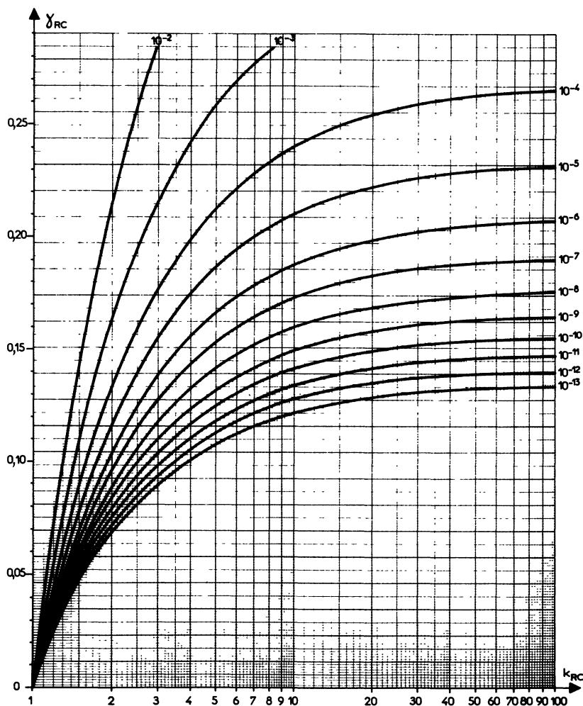
Figure. 1 – Probabilité de défaillance en fonction du coefficient de sécurité k_{RC} et du coefficient de variation \gamma_{RC} (cas de deux lois normales)
