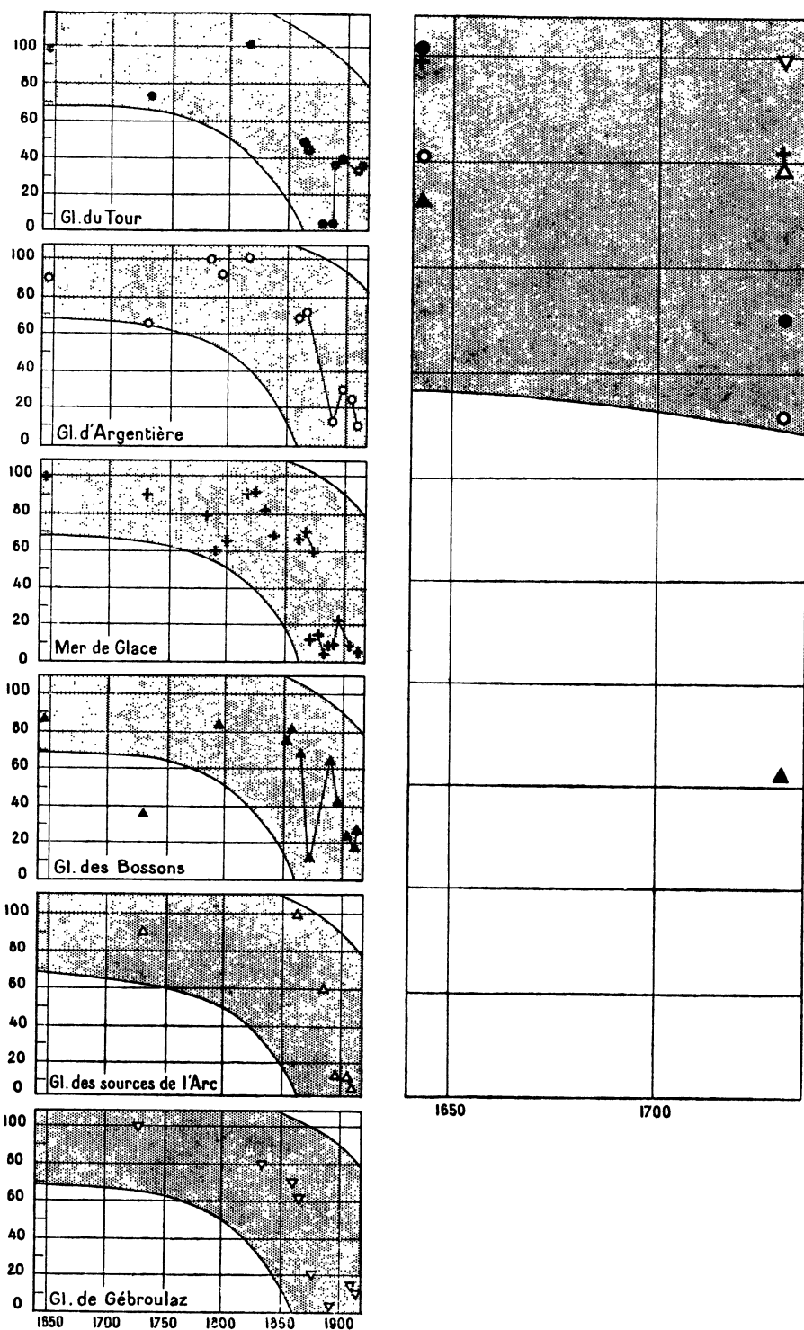
Graphique 3 : La longue durée : les glaciers de Savoie
