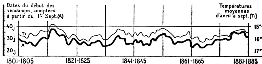
Graphique 1 - Dates de vendanges et températures (moyennes mobiles quinquennales).
