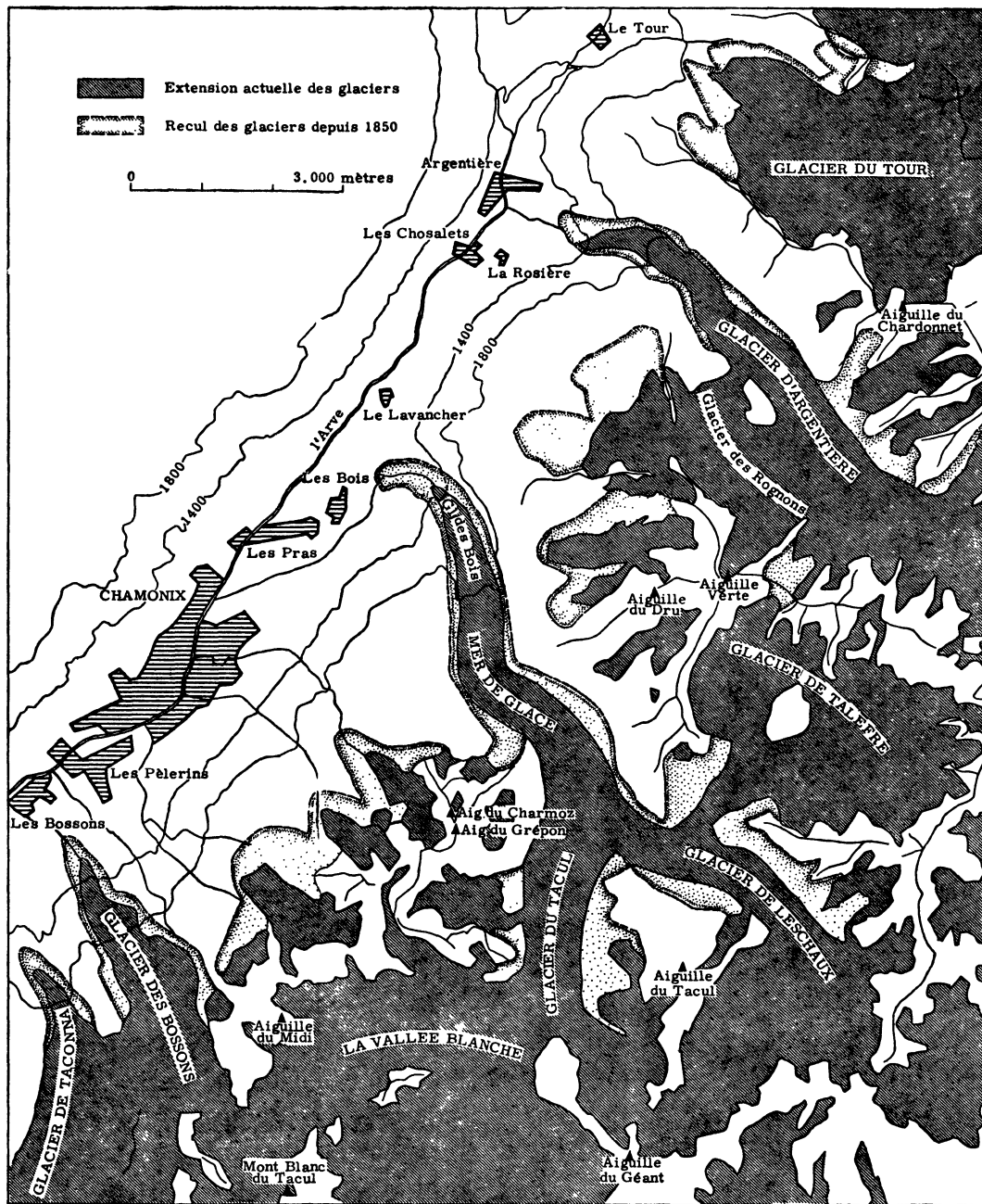
Graphique 4 : Les glaciers de Savoie
