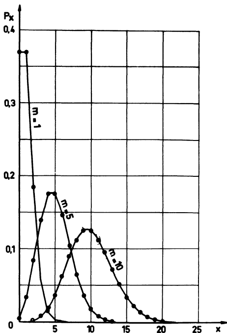
Figure 1 Représentation de lois de Poisson de moyennes 1, 5 et 10.
