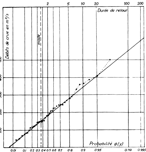
Fig. 84. - Durance à l'Archidiacre. Crues d'automne 1916-1955 (Loi de Fréchet).
