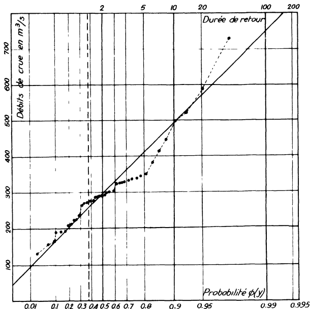
Fig. 71. - Durance à l'Archidiacre. Crues de printemps 1916-1955 (Loi de Gumbel).
