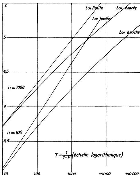
Fig. 1.- Loi de la plus grande de n = 100 et n = 1.000 variables normales
