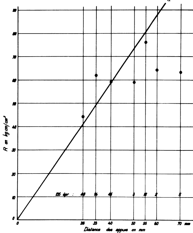
Graphique n° 8 - Résilience à + 15 °C d'où \text{FRAGILITE} = \frac{R}{d} = 14,5 \text{ kgcm/cm}^3
