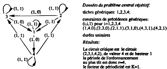
Figure 5. — Graphe bivalué associé au problème central répétitif.
