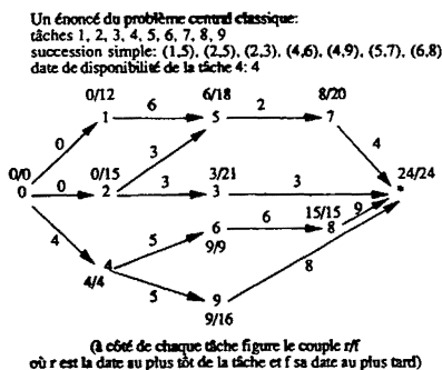
Figure 2. — Le graphe potentiel associé.
