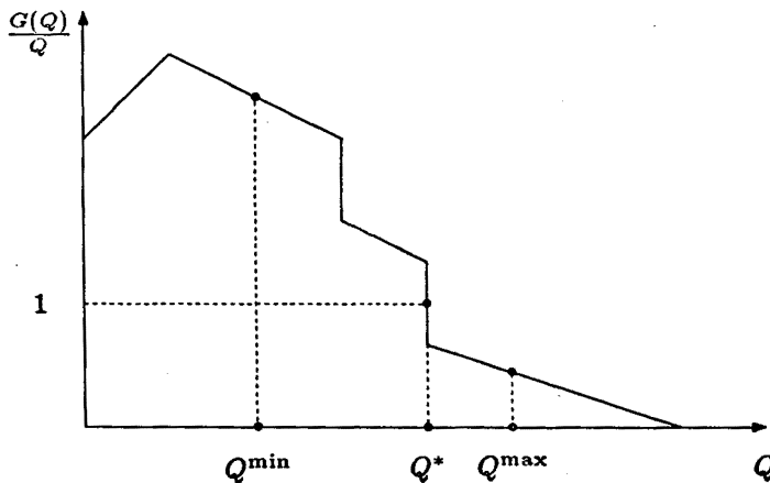
Figure 1. — La fonction de production globale.
