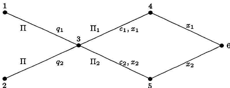
Figure 2. — Un exemple de demande dérivée.
