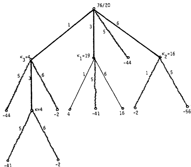
Figure 1. — Arborescence due à l'application de la méthode du simplexe inverse à l'exemple PL2. Arcs — : solutions de la première phase; arcs - - - : solutions de la seconde phase; arcs . . . : solutions multiples déjà calculées en première phase.
