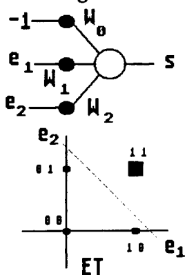
Fig 6. Le ET logique est linéairement séparable.
