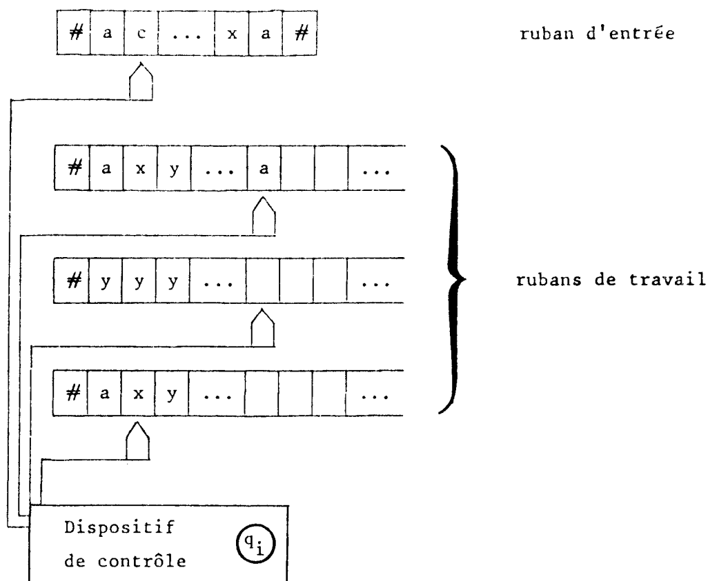
Fig. Une machine de Turing à 4 rubans
