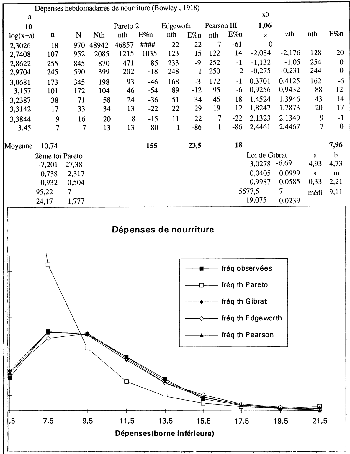
Figure 2. Comparaison d'ajustements sur dépenses de nourriture.
