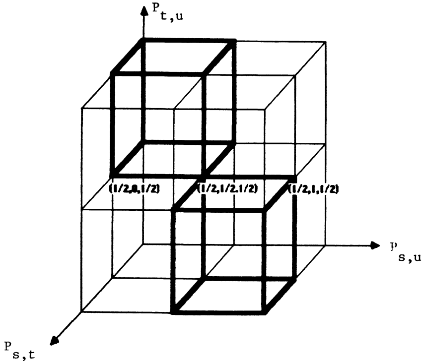
Figure 2 : Géométrie de l'espace des paramètres pour le test statistique de la transitivité faible, dans le cas de trois objets. Les deux demis cubes délinéés en gras représentent le complément de l'hypothèse nulle.
