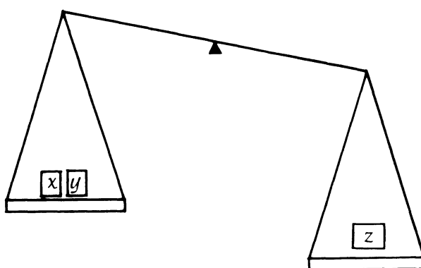
Figure 1 : Mesurage fondamental des poids par la balance à deux plateaux. La situation de la figure est notée x * y \lesssim z
