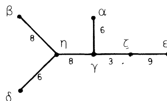
Figure 10. L'arbre A minimum pour D .
