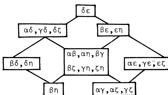
Figure 8. La préordonnance R_7
