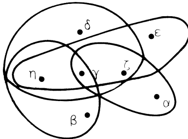
Figure 3. La famille de parties \{F_1, F_2, F_3, F_4\}
