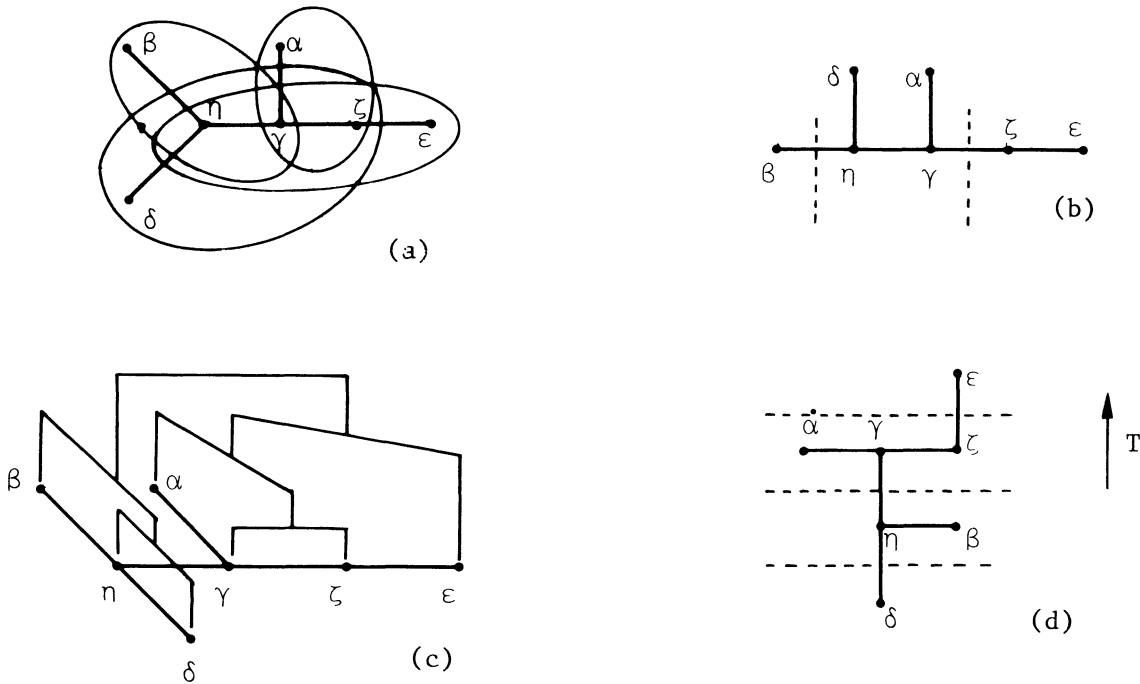
Figure 11. L'arbre A est compatible avec chacune des structures \mathcal{F} , T , \Pi et H sur X .
