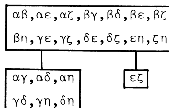
Figure 4. La préordonnance R_5
