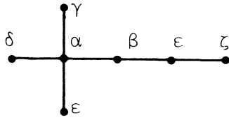
Figure 5. L'arbre A_5
