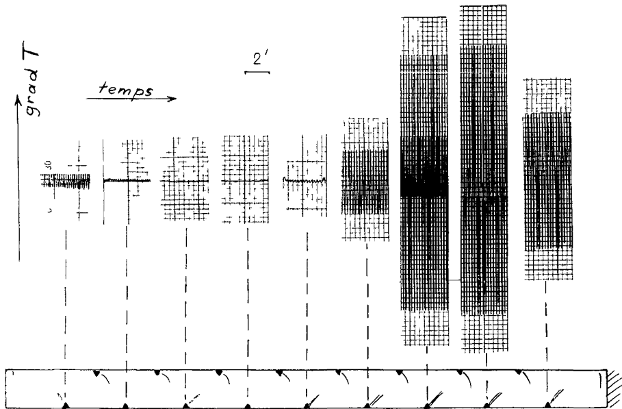
Un exemple de comportement très hétérogène de la chaîne de rouleaux. On a représenté quelques minutes d'enregistrement de la variation temporelle d'un gradient de température, relevé dans chaque longueur d'onde. La coexistence de régions oscillantes et non oscillantes est frappante.
