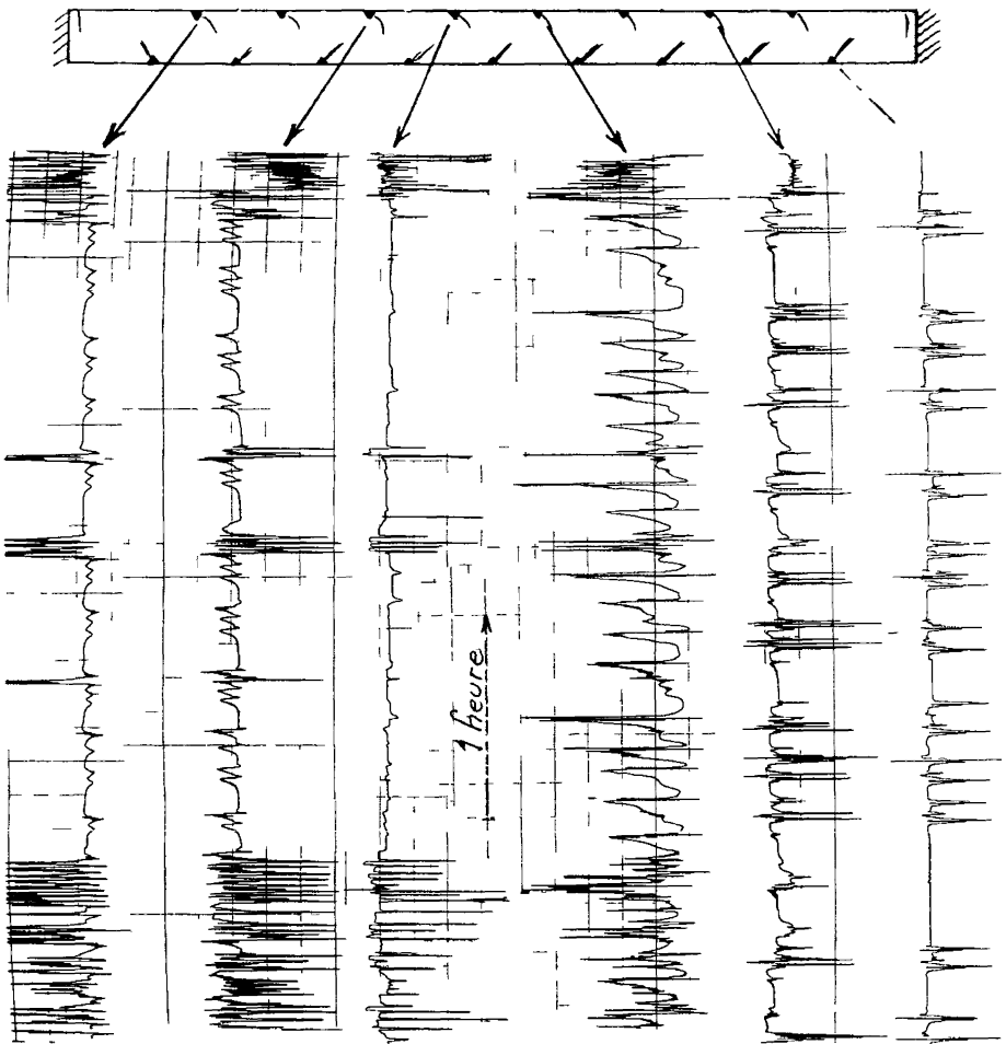
Evolution temporelle des gradients thermiques mesures en diverses positions de la chaîne de rouleaux. On notera la présence de bouffées survenant erratiquement et à des moments différents selon les emplacements considérés.
