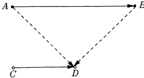
Figure 2. – Une exécution n'admettant pas de modèle temps global.
