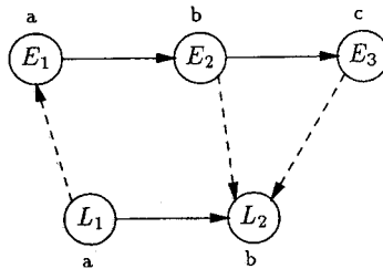
Figure 9. – Exécution atomique mais non régulière.
