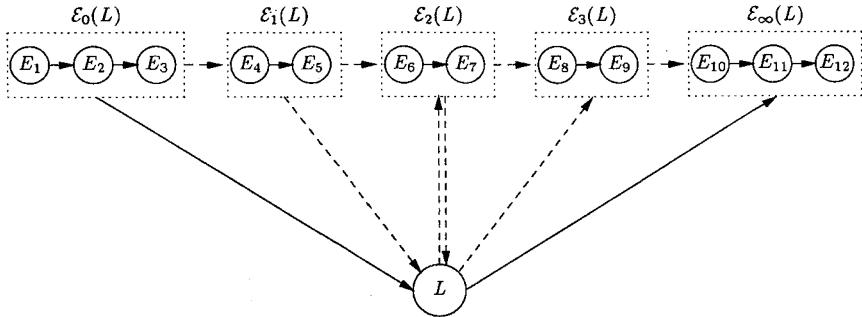
Figure 3. – Partition d'une suite d'écritures par une lecture
