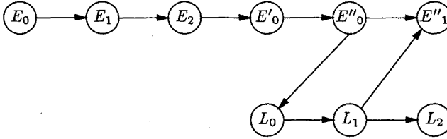
Figure 8. – Implémentation incohérente d'un registre à m valeurs.
