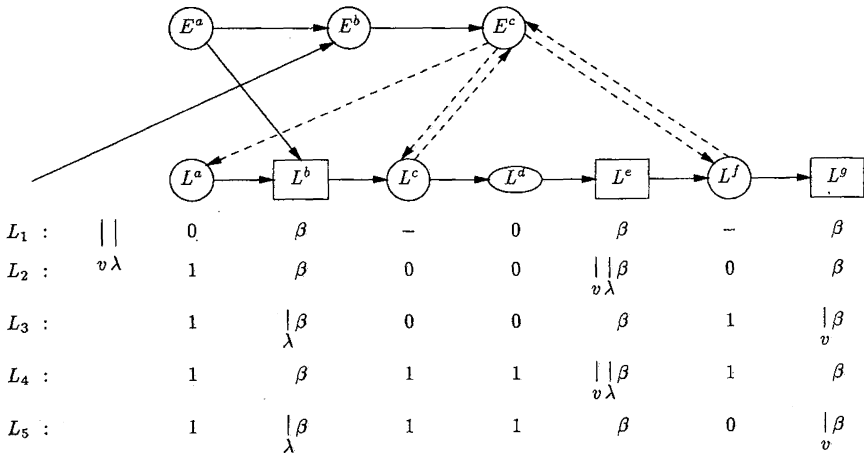
Figure 12. – Un exemple d'exécution.
