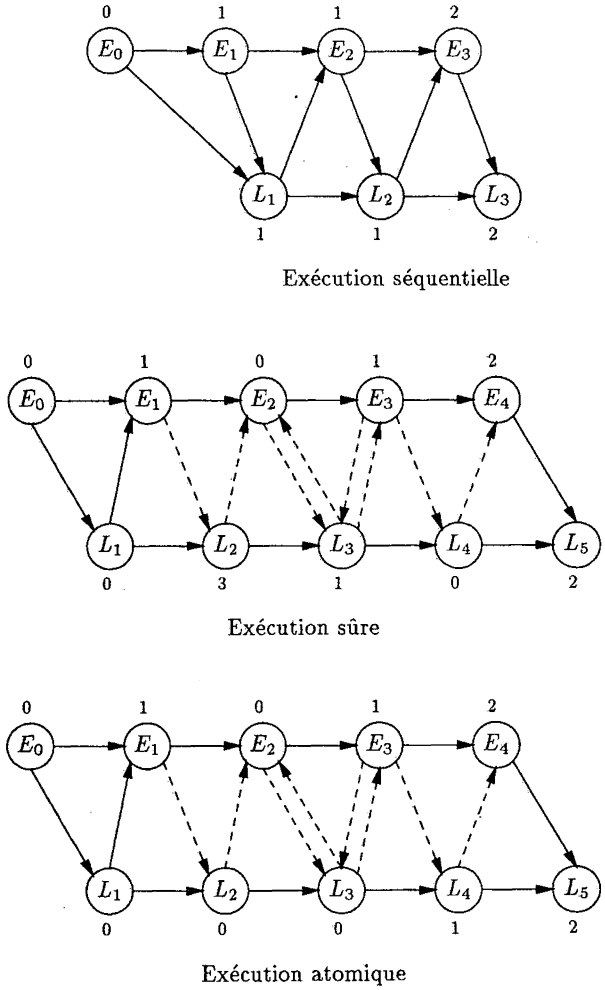
Figure 4. – Exécutions séquentielles, sûres et atomiques, les valuations sont indiquées par un nombre situé à côté de chaque action.
