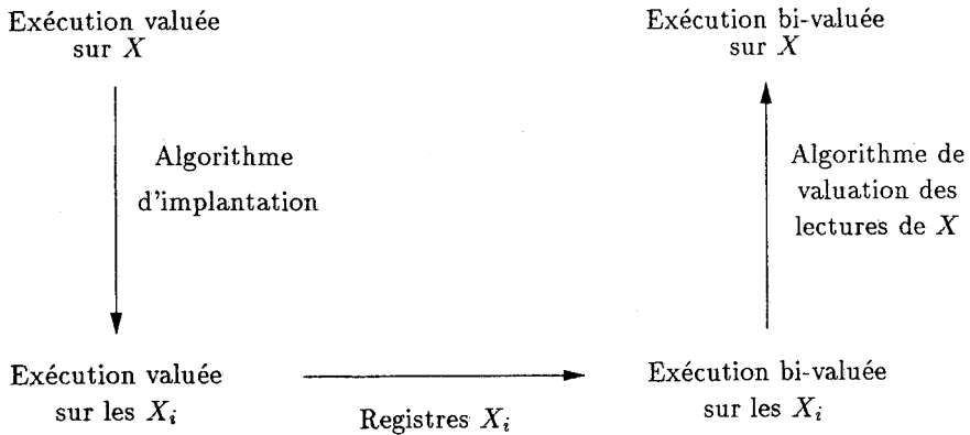
Figure 5. – Schéma d'une réalisation.
