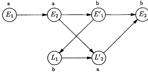
Figure 6. – Exécution non atomique d'un registre multi-lecteur.
