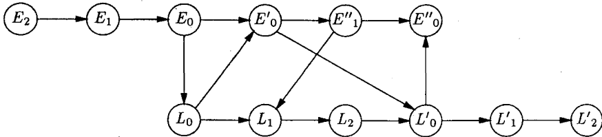
Figure 7. – Exécution non atomique d'un registre à k valeurs.
