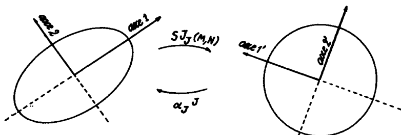
Figure : Système orthogonal Rep transformé par S_J^J(M,N) en un système orthogonal Rep' : pour plus de clarté on a translaté la sphère Sph relativement à l'ellipsoïde Ell ; on notera que dans le cas de la figure, les deux systèmes orientés Rep et Rep' ne sont pas de même sens : donc \alpha_J^J (qui envoie l'axe orienté 1' sur l'axe orienté 1 ; et de même 2' sur 2) est ici une isométrie inverse.
