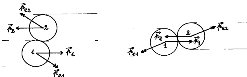
Figure 4-1: Deux cas de chocs entre deux sphères. À gauche, choc périphérique : faible transfert de quantité de mouvement. À droite, choc quasi-central : les deux sphères rebroussement chemin en échangeant presque toute leur quantité de mouvement.
