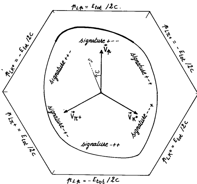
Figure 4-5 Diagramme hexagonal de Van Hove pour la réaction K^+ p \rightarrow p^+ \pi^+ K^0 . Énergie du K^+ incident dans le système lié au laboratoire = 3 GeV ; énergie totale dans un système lié au centre de gravité : E_{\text{tot}} = 2,56 GeV ; dans ce système l'axe des p_L est orienté pour que le proton incident ait un moment positif \approx 1,04 GeV/c. Le plan est divisé en six angles égaux correspondant chacun à une signature : e.g. ++ : p_{Lp} > 0 ; p_{L\pi^+} < 0 ; p_{LK^0} > 0 . On a représenté la frontière du domaine des triplets permis, ainsi que la frontière de l'hexagone : \sum |p_{Lej}| = E_{\text{tot}} ; e.g. l'arête de signature +- de cet hexagone a pour équation p_{Lp} = E_{\text{tot}}/2c ; p_{L\pi^+} + p_{LK^0} = -E_{\text{tot}}/2c . Dans le système du laboratoire la vitesse de recul du proton a pour minimum 0,02c, sur la frontière du domaine des triplets permis on a renforcé l'arc sur lequel v_{pL} \leq 0,2c .
