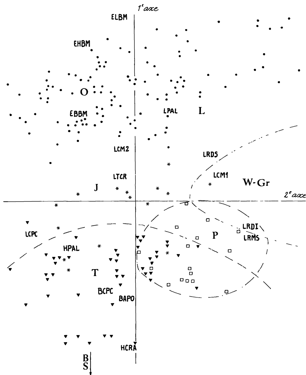
Plan 1-2 de l'analyse pondérée : les individus des quatre espèces O, T, J, P (O: C. occidentalis ; T: C. theresae ; J: C. jouvenetae ; P: C. poensis ) sont pondérés par l'inverse de l'effectif de leur espèce ; on les a représentés par les sigles : • (O) ; ▼ (T) ; * (J) ; □ (P) . la lettre L indique la place des C. lamottei ; on a esquissé par leurs contours les domaines (empruntés sur ce plan) des espèces T et P, ainsi que le domaine approximatif W-Gr de l'espèce C. wimmeri et groupes adjacents très peu représentés dans l'échantillon ; une flèche signale les espèces C. bottegii et Sylvosorex m. très écartées à l'extrémité inférieure de l'axe .
