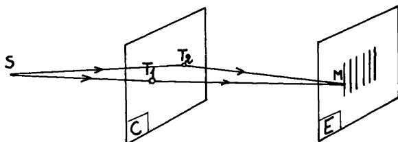
Figure 3-6 : Schéma des interférences obtenues par les trous d'Young
