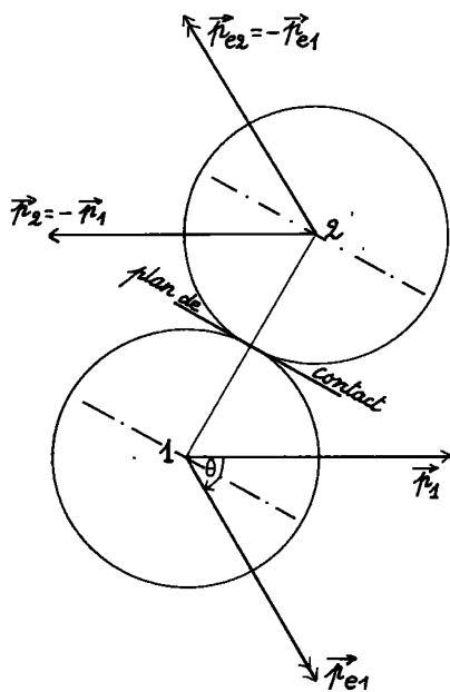
Figure 3-1 a et b : ci-dessous, a, représentation schématique des deux faisceaux opposés, avec un exemple de choc ; ci-dessous, b, détail de la description cinématique d'un choc élastique entre deux sphères égales
