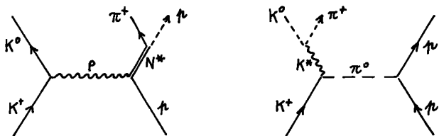
Figure 3-5 : graphes de Feynman pour deux sous-canaux de la réaction : K^+ + p \rightarrow K^0 + \pi^+ + p à gauche : K^+ + p \rightarrow K^0 + N^* \rightarrow K^0 + \pi^+ + p ; à droite : K^+ + p \rightarrow K^* + p \rightarrow K^0 + \pi^+ + p .
