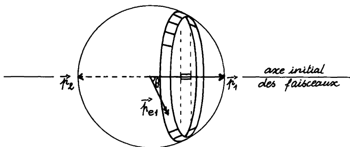
Figure 3.2 : Sur la sphère S des événements permis, on a représenté une zone hachurée où \theta est constant à d\theta près ; l'aire, ou masse de cette zone est proportionnelle à la largeur |d \cos \theta| = |\sin \theta d\theta| de sa projection sur l'axe initial des faisceaux.
