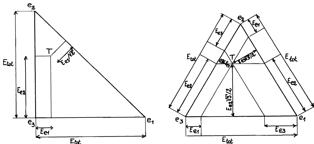
Figure 3-3 : deux variantes de la représentation des énergies de trois particules émergentes en coordonnées triangulaires ; à gauche, triangle isocèle et rectangle ; à droite, triangle équilatéral. Ici, symétrie parfaite entre les particules ce qui est notamment recherché si celles-ci ont même masse ; là, des coordonnées rectangulaires usuelles pour deux énergies.
