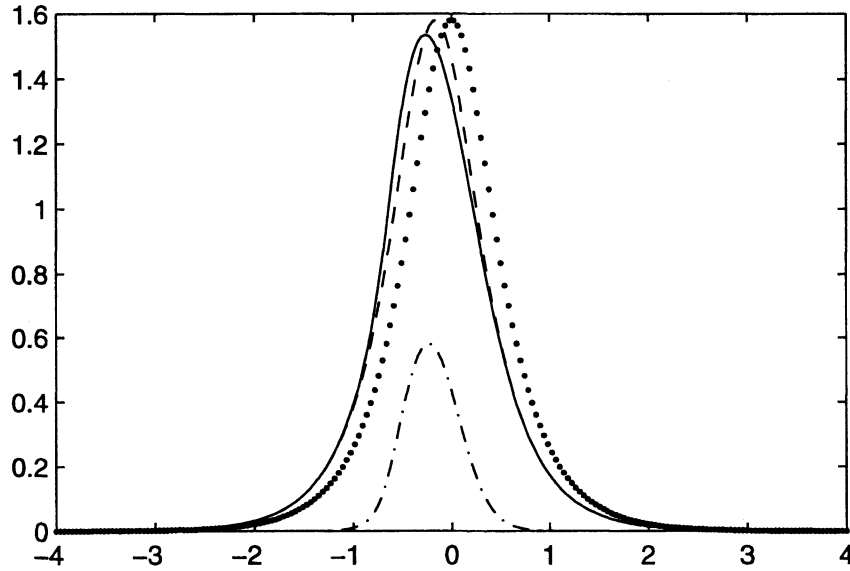
Fig. 2: |q_o| (dotted ..), |q(t_{max})| (continuous line -), |q_A(t_{max})| (dashed -) and |q(t_{max}) - q_A(t_{max})| (dashed-dotted .-) for: \epsilon = 0.025 , t_{max} = 0.088 , \Delta x = 0.04 , \Delta t = 16.10^{-5} , [a; b] = [-4; 4] , \Delta_\epsilon = 0.36 .
