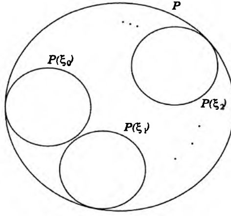
FIG. 4: Chaque bout \mathcal{P} d'une composante analytique de \mathcal{E}(R) a une infinité de disques de Siegel attachés.
