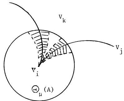
Figure 3 : Le voisinage P est hachuré selon ses rayons. La longueur de ces derniers tend vers 0 au voisinage de V_i .
